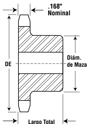
Largo Total Tipo B
