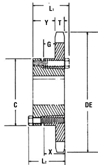
Buje QD — Tipo B
