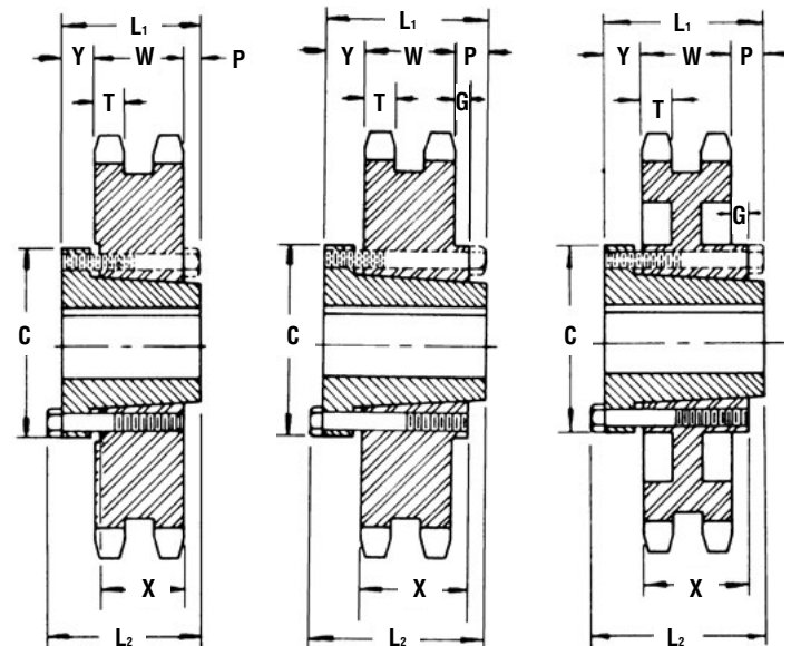
Buje QD Tipo C 1
