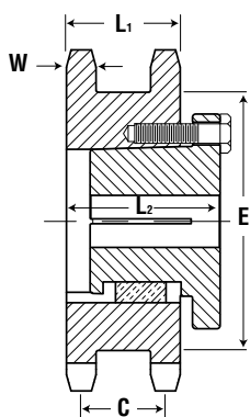
Buje MST® Tipo B
