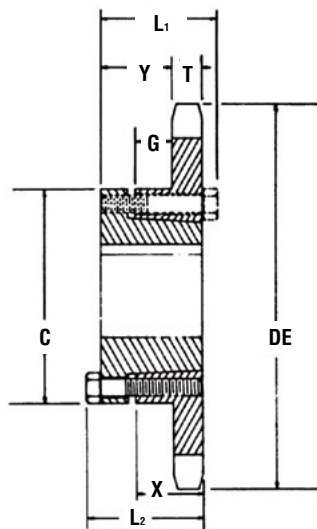
Tipo B Buje QD
