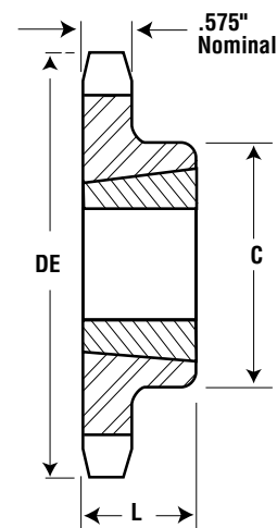
Tipo B Buje Taper
