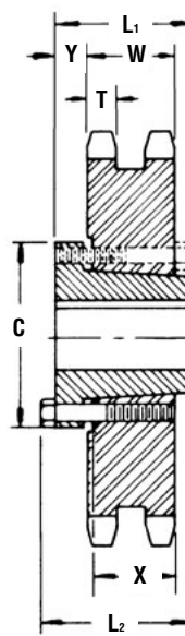
Buje QD Tipo C 1
