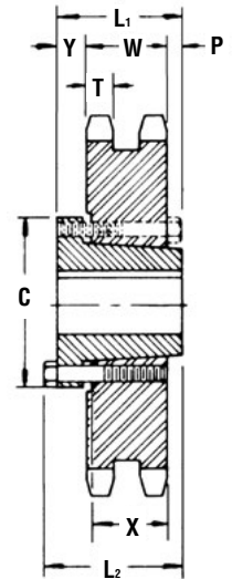
QD — Tipo C
