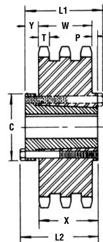
Tipo C Buje QD
