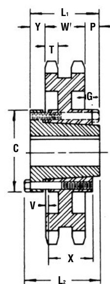
Buje QD Tipo C 6
