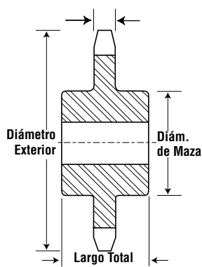
Sencillo Tipo C
