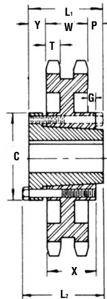
Buje QD Tipo C 5
