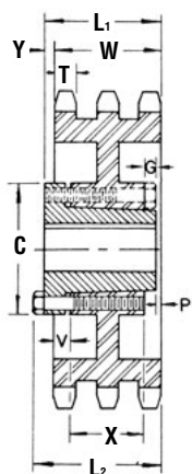
Tipo B 1 Buje QD
