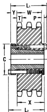
QD - Tipo C
