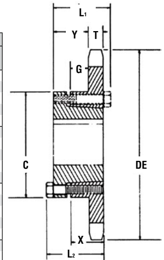
Buje QD — Tipo B
