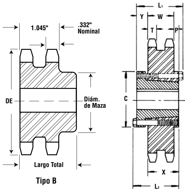
Buje QD Tipo C
