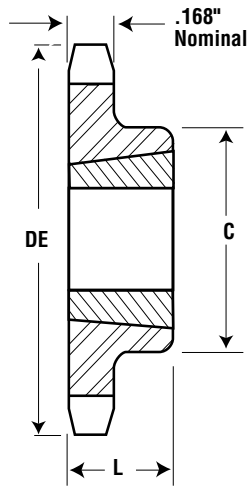
Tipo B Buje Taper
