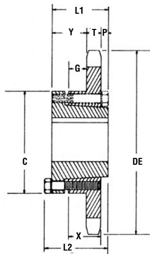
Tipo B 1 Buje QD
