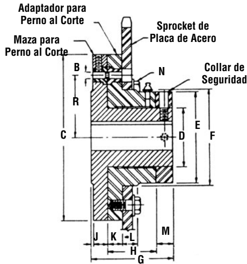
Dimensiones del Ensamble de Perno al Corte (Pulgadas)
