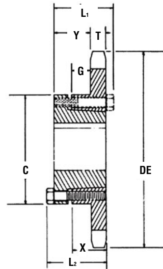
Tipo B Buje QD
