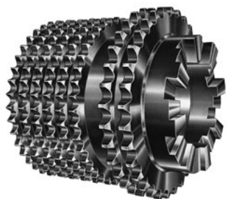
Sprockets de Hileras Múltiples para Aplicaciones Petroleras con Mordazas de Embrague
