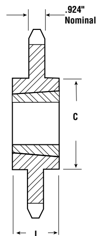
Tipo C Buje Taper
