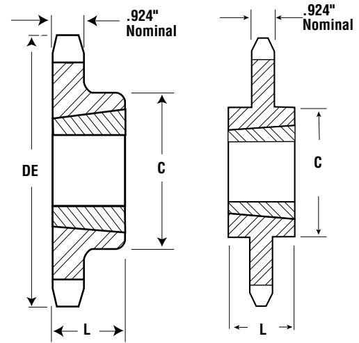
Tipo B Buje Taper
