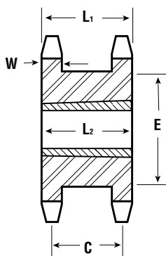
Buje Taper Tipo A
