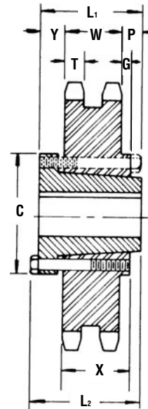
Buje QD Tipo C 2
