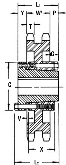
Buje QD Tipo C 6
