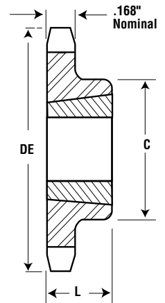
Tipo B Buje Taper
