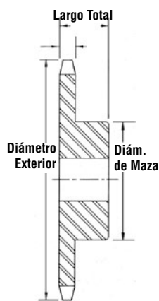
Sencillo Tipo B
