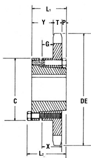
Tipo B 1 Buje QD
